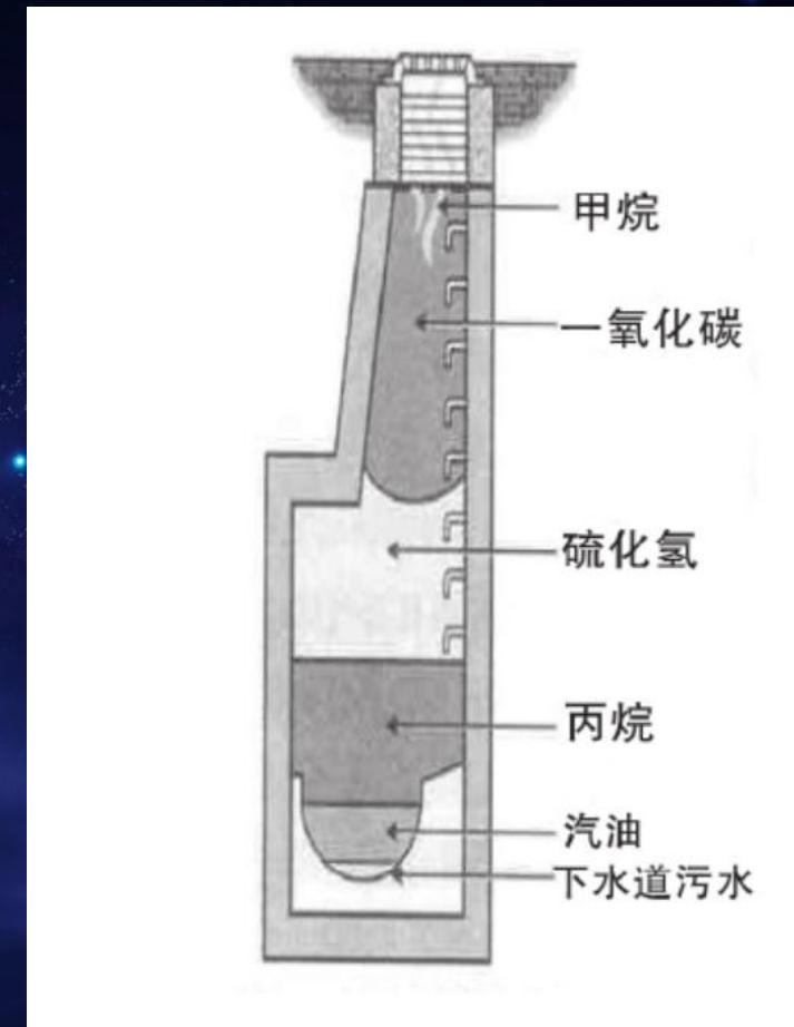
下水道检修井不同气体聚集位置
