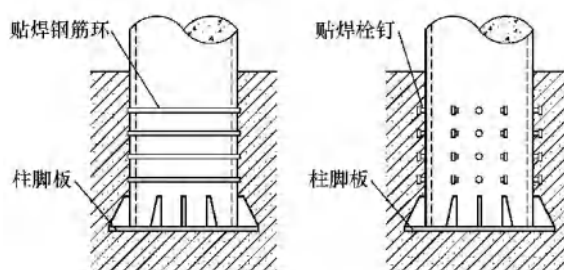
图2 插入式柱脚
