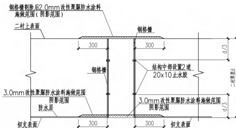
图 17 钢筋格栅穿防水层构造剖面图
