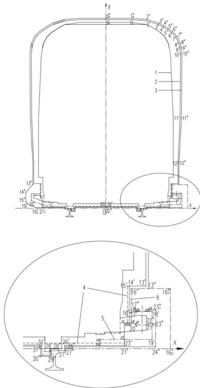
图 B.0.1-3 B 1 型 DC1500V 下部受流车区间车辆限界和区间直线地段设备限界
