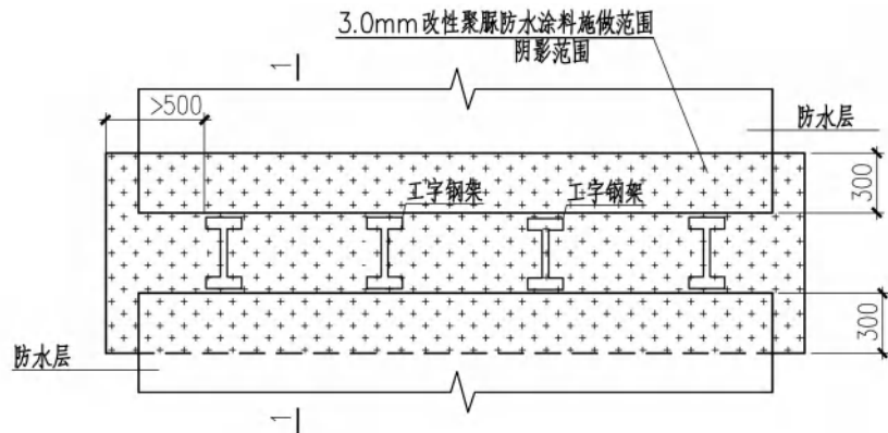
图 18 型钢格栅穿防水层构造平面图
