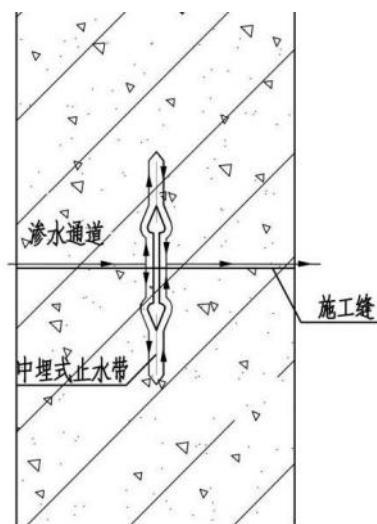
图 20 中埋式止水带防水原理图配图
