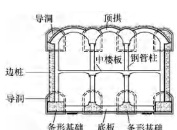
图 6 洞柱逆作法
