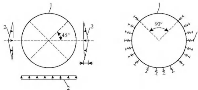
(a) 假定抗力法 (b) 地基弹簧法（局部弹簧模式）
