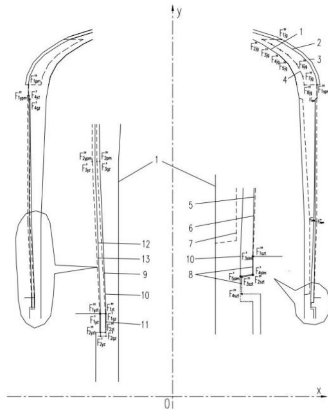
图 C.0.1-2 B 2 型车计算站台长度范围内附加车辆限界、直线站台及站台屏蔽门限界、检修库高低平台限界
