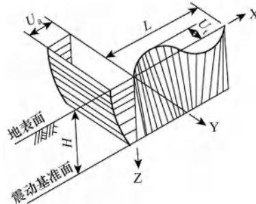
图 12.8.6 假定地层变位法地层沿深度及水平方向的变形模式
