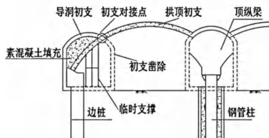
图7 拱部作法示意图
